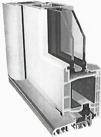
normál szárny (8081/8078)
