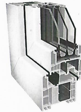
Normál szárny (6079)
