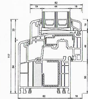
LUMAXX szárny (6055)
