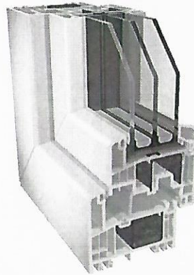
Normál szárny (6079)
