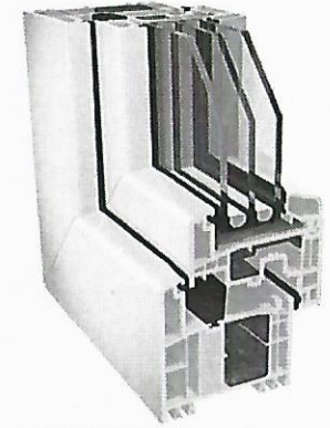
LUMAXX szárny (6055)
